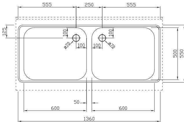
Boven aanzicht
